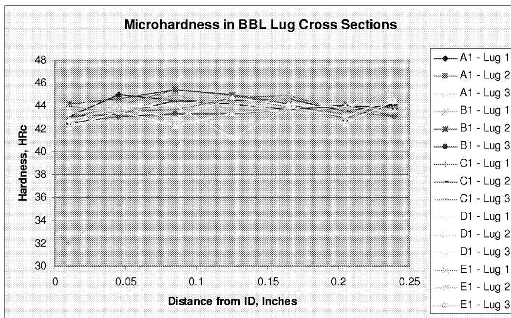
Figure 7: Locking Lug Microhardness Data.
